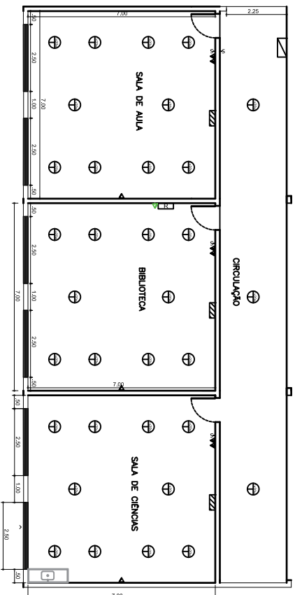
PLANTA BAIXA (PROJETO ELÉTRICO/HIDROSSANITÁRIO) ESC.1:100
