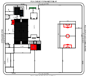
LOCALIZACAO COBERTURA ESC: 1:100
