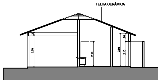
CORTE ESC. 1:100
